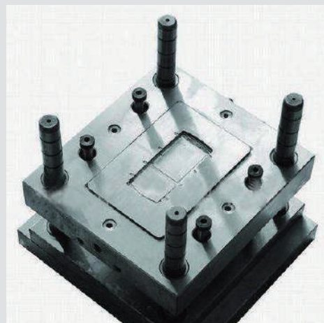
ダイホルダ
