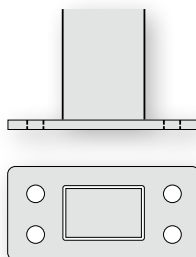
Rechteck-Steher 60x40 mm mit verschweißter Montageplatte 4-Loch
